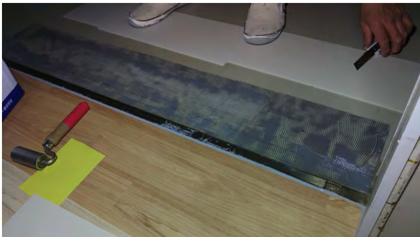
居室段差調整板 取付状況 2024. 3. 28~29
